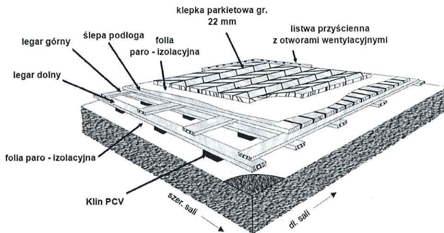
Rys. 1 – Przekrój podłogi sportowej
